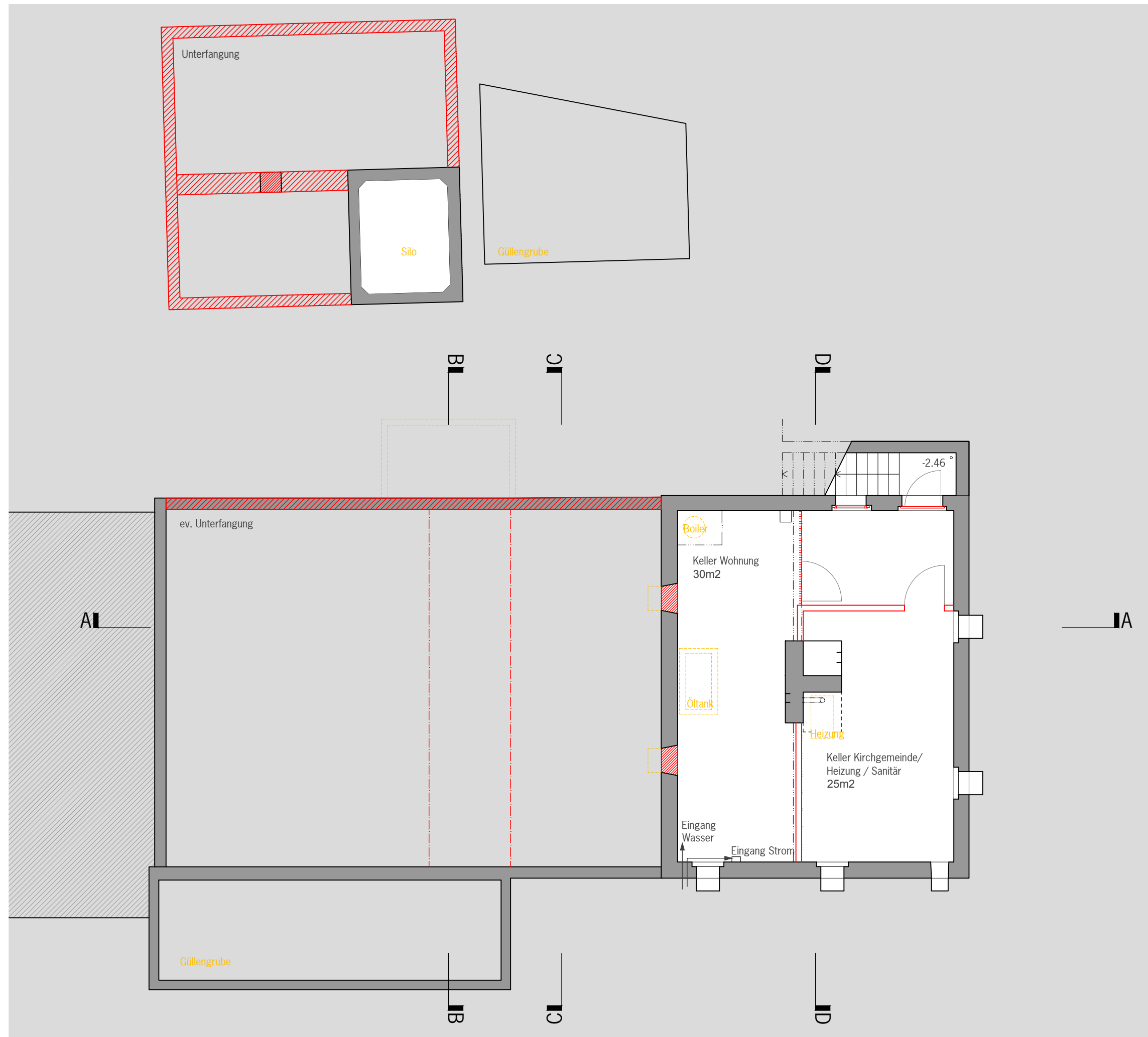
Grundriss UG
