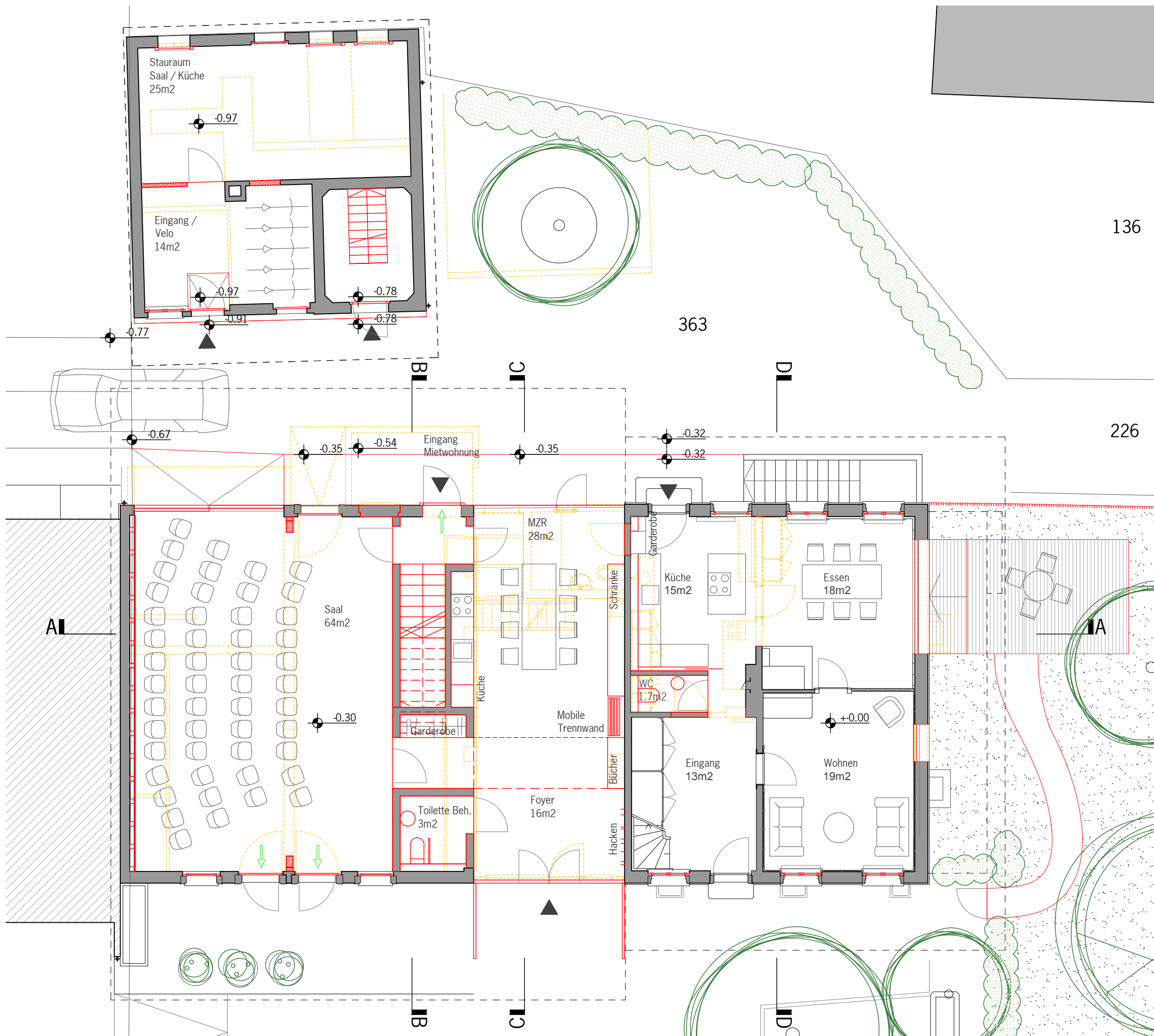
Grundriss EG
