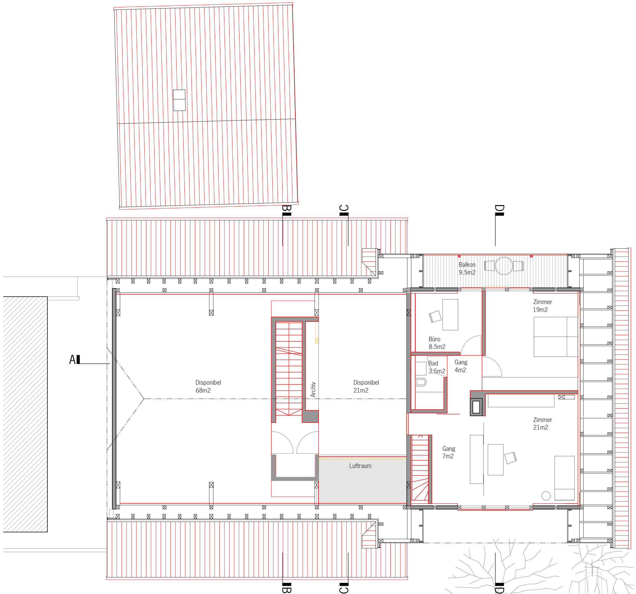
Grundriss DG
