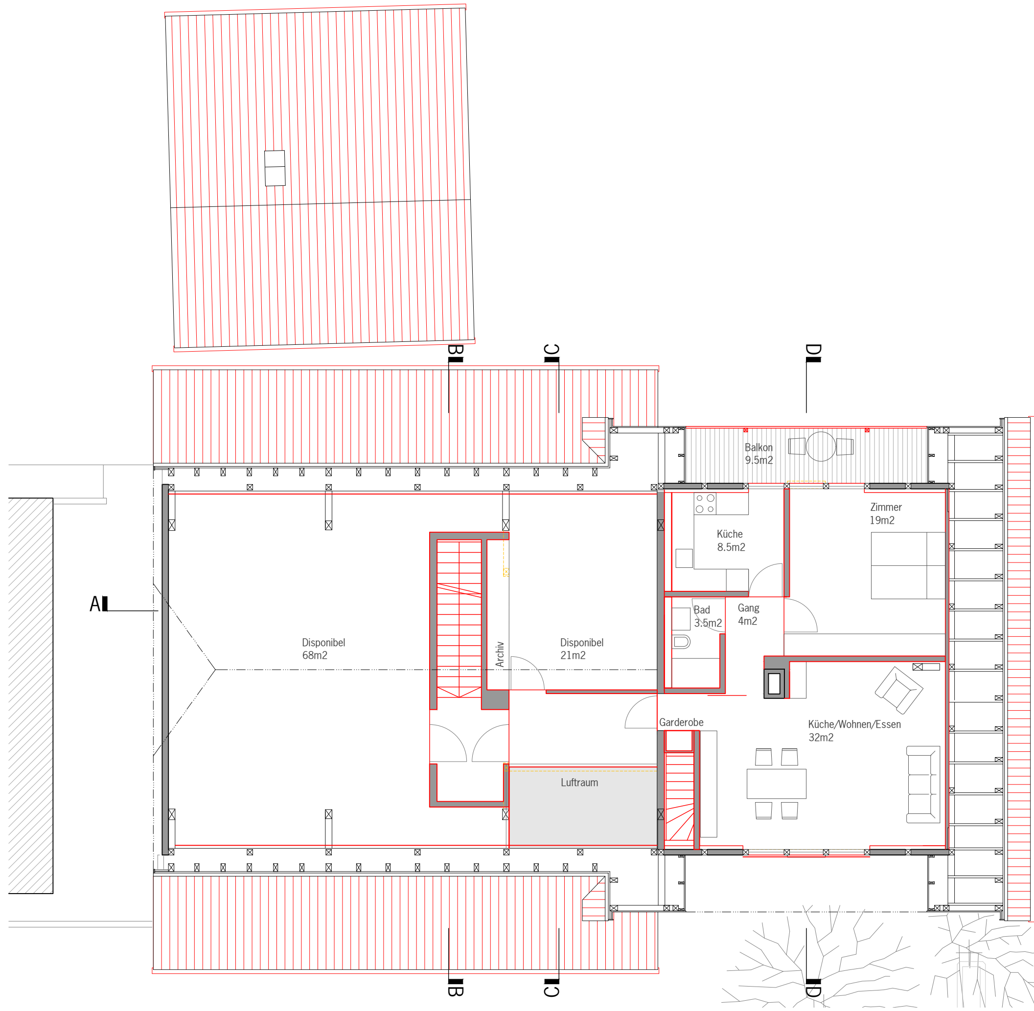
Grundriss DG- getrennte Wohnung
