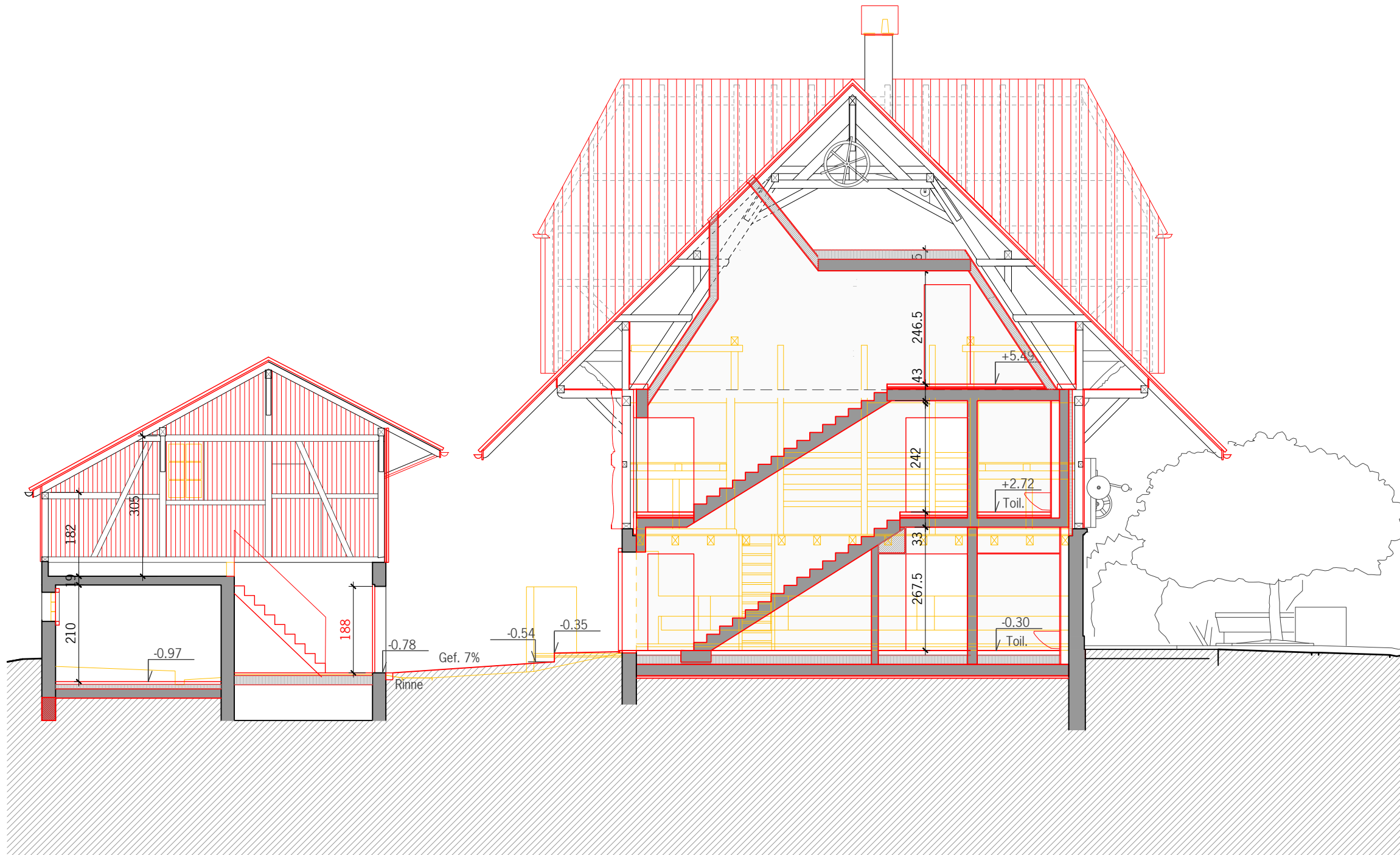
Schnitt BB
