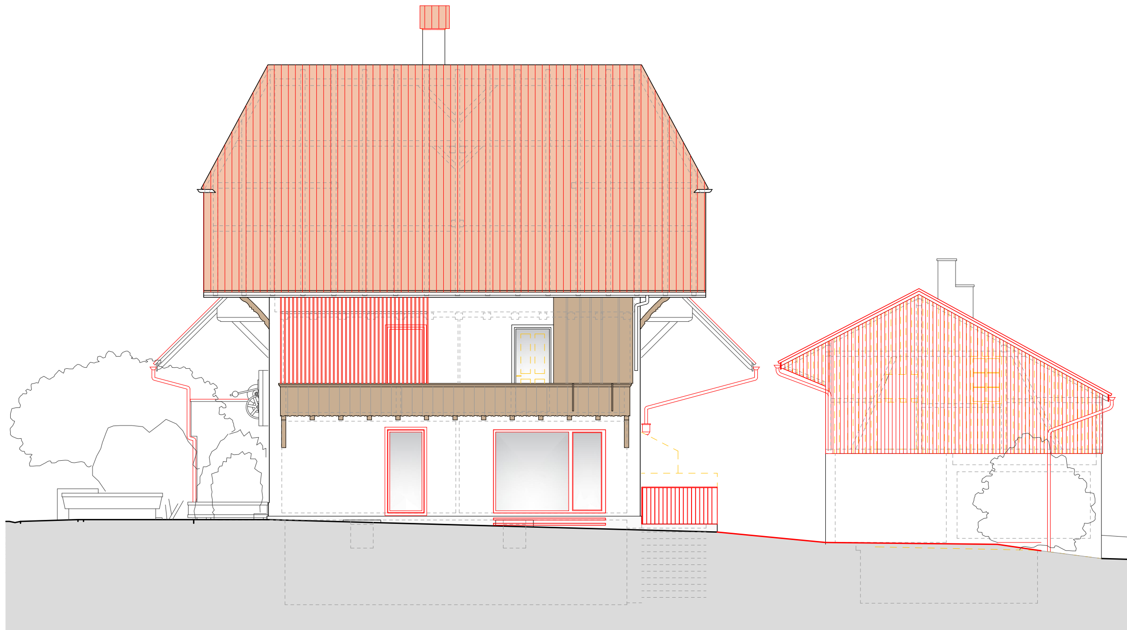
Fassade Nord-Ost
